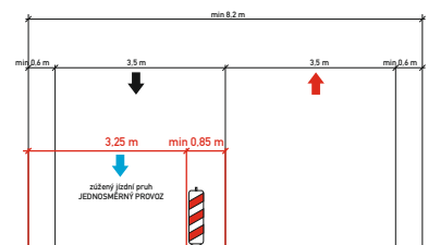
Příčný řez místem stavby
