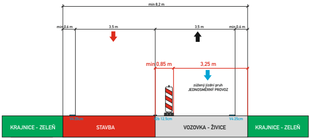
Příčný řez místem stavby
