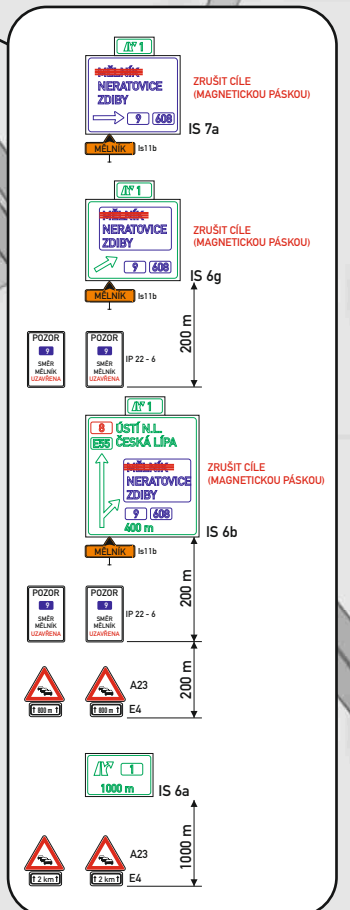
Detail značení na dálnici D8 PS před Exitem 1
